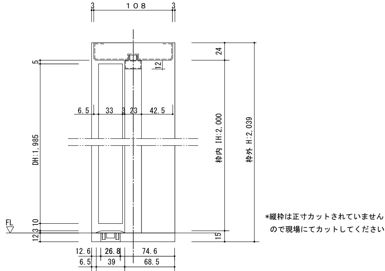
断面図
