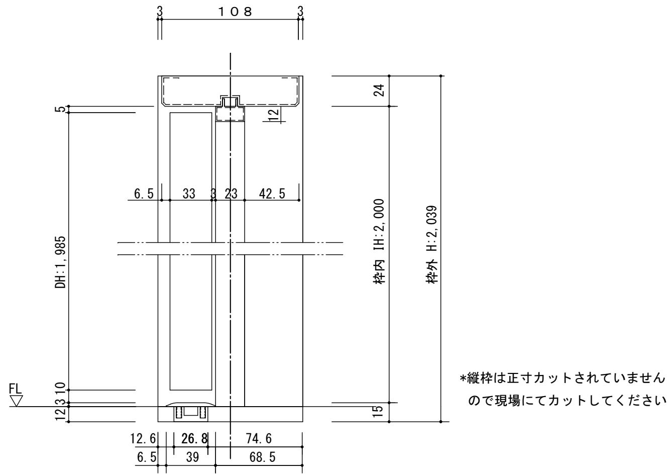
断面図
