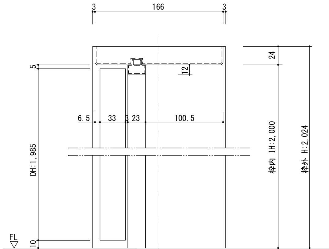
断面図
