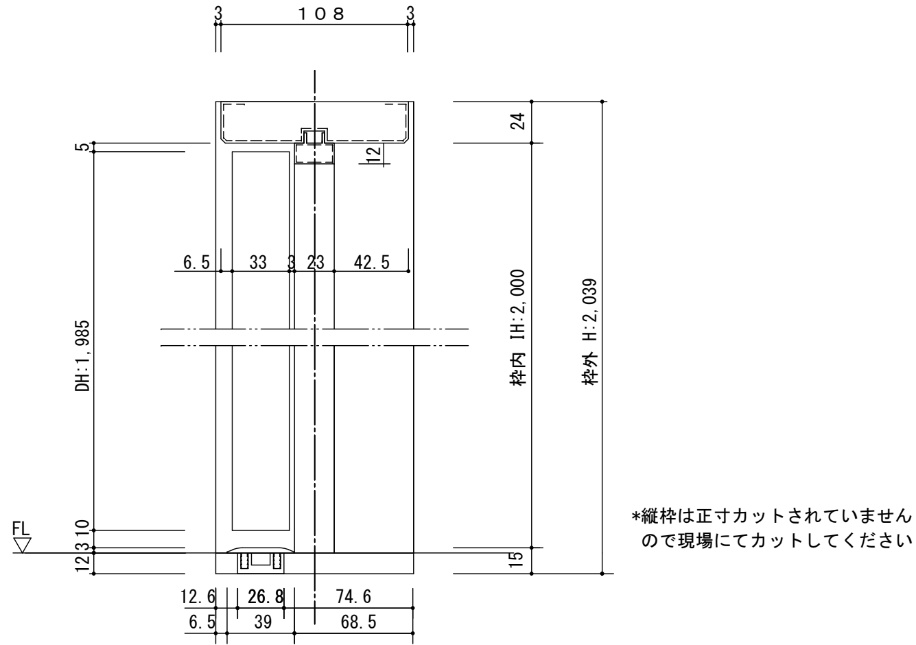
断面図
