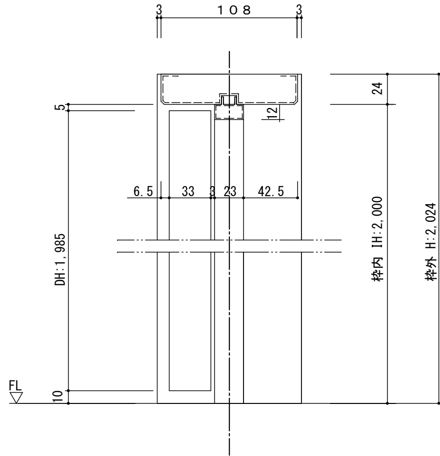
断面図
