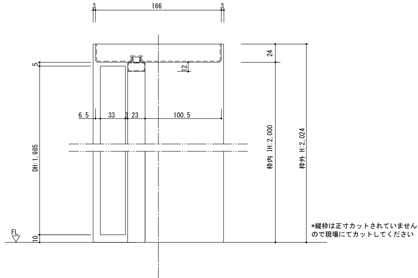
断面図
