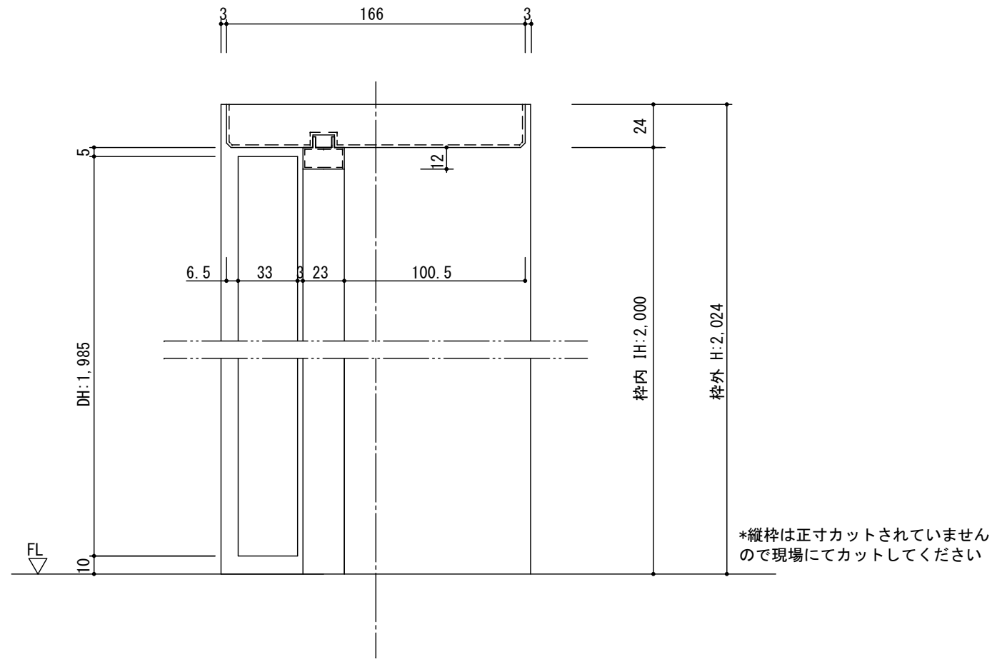
断面図
