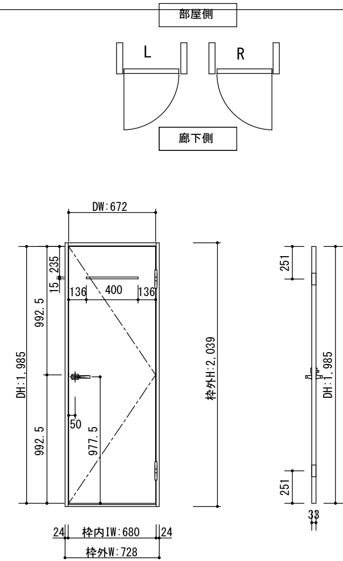
正面図
