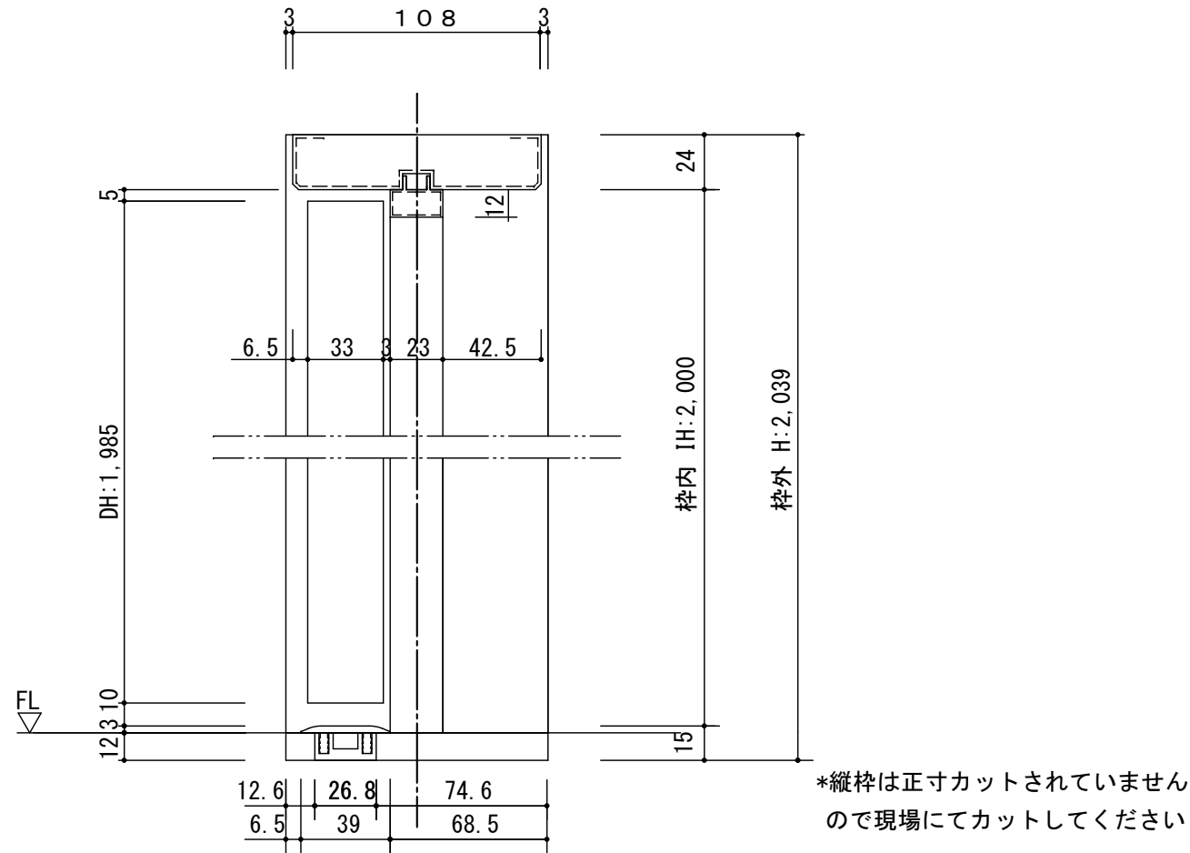
断面図
