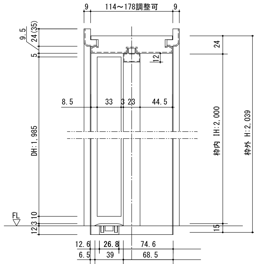
断面図
