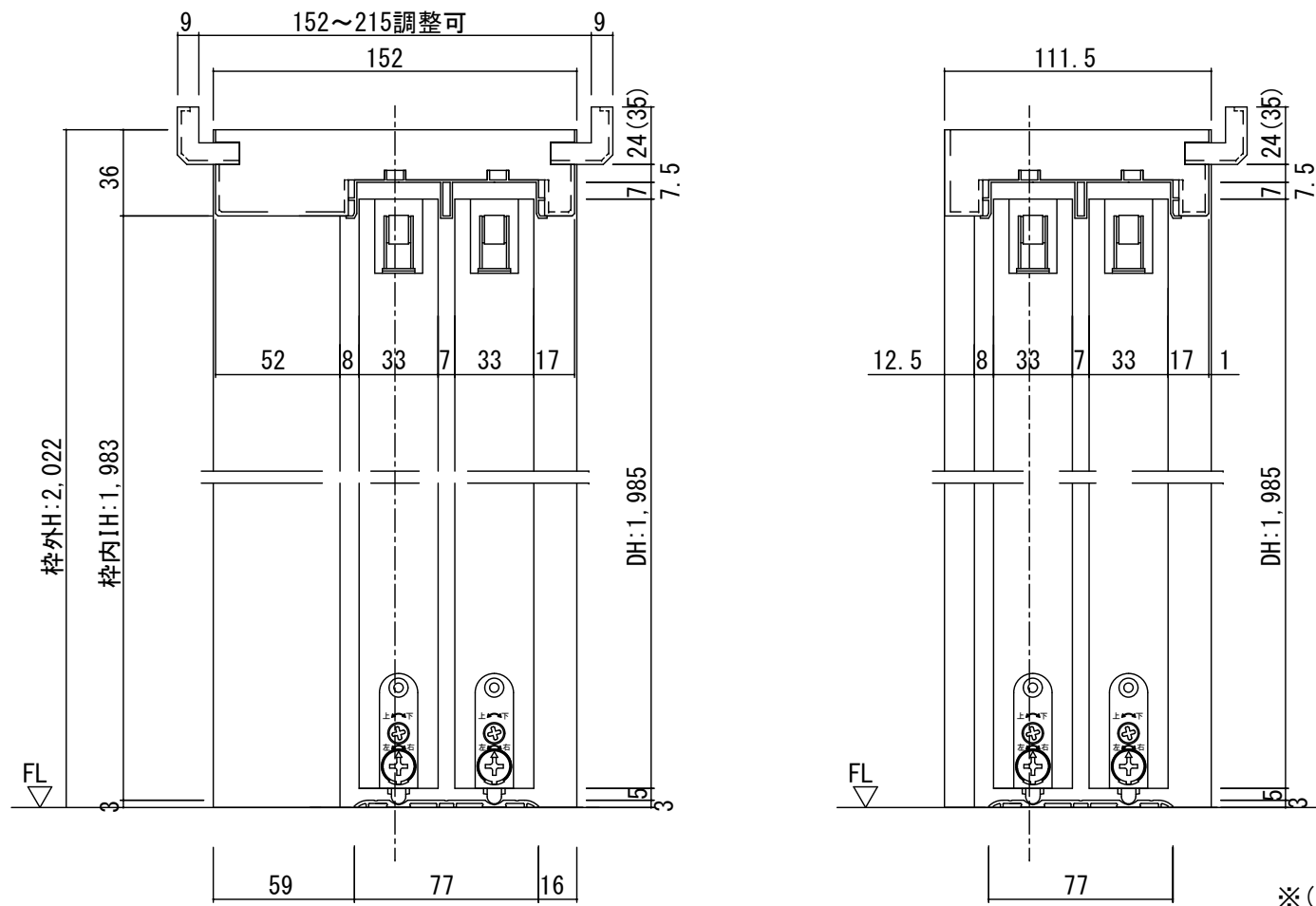
断面図
