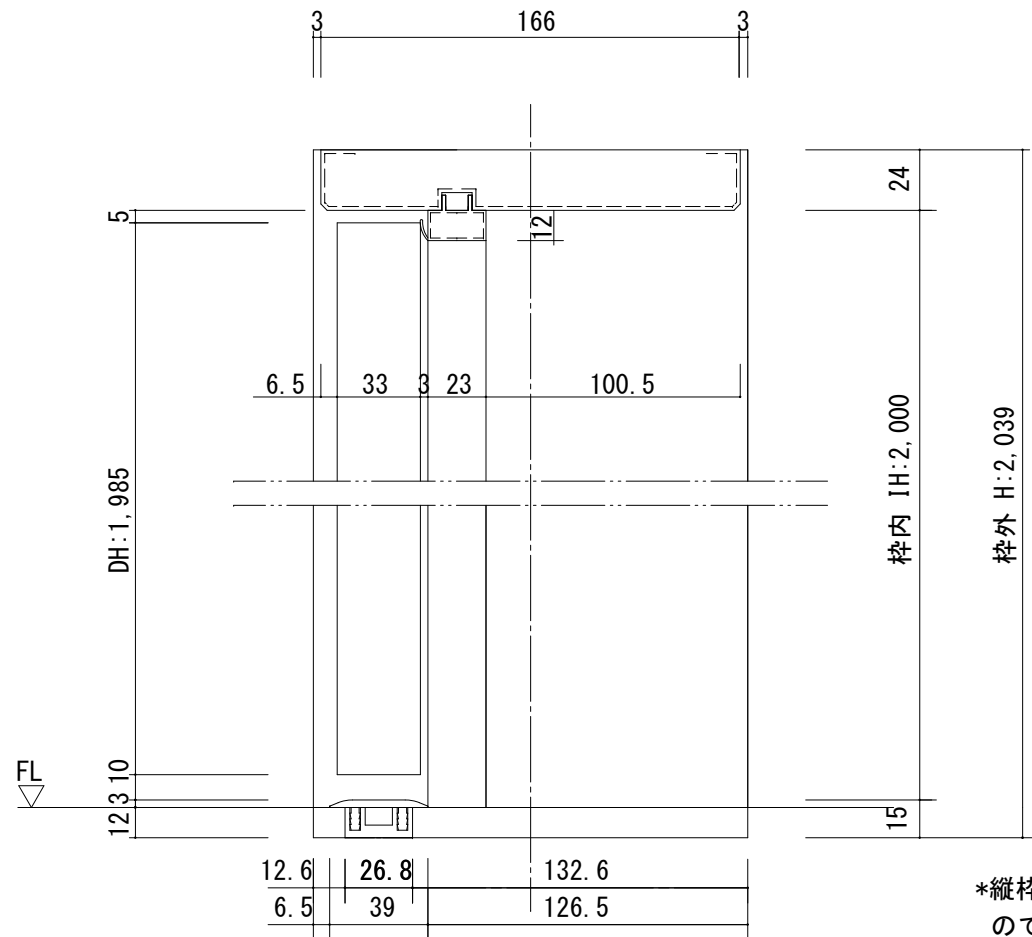
断面図
