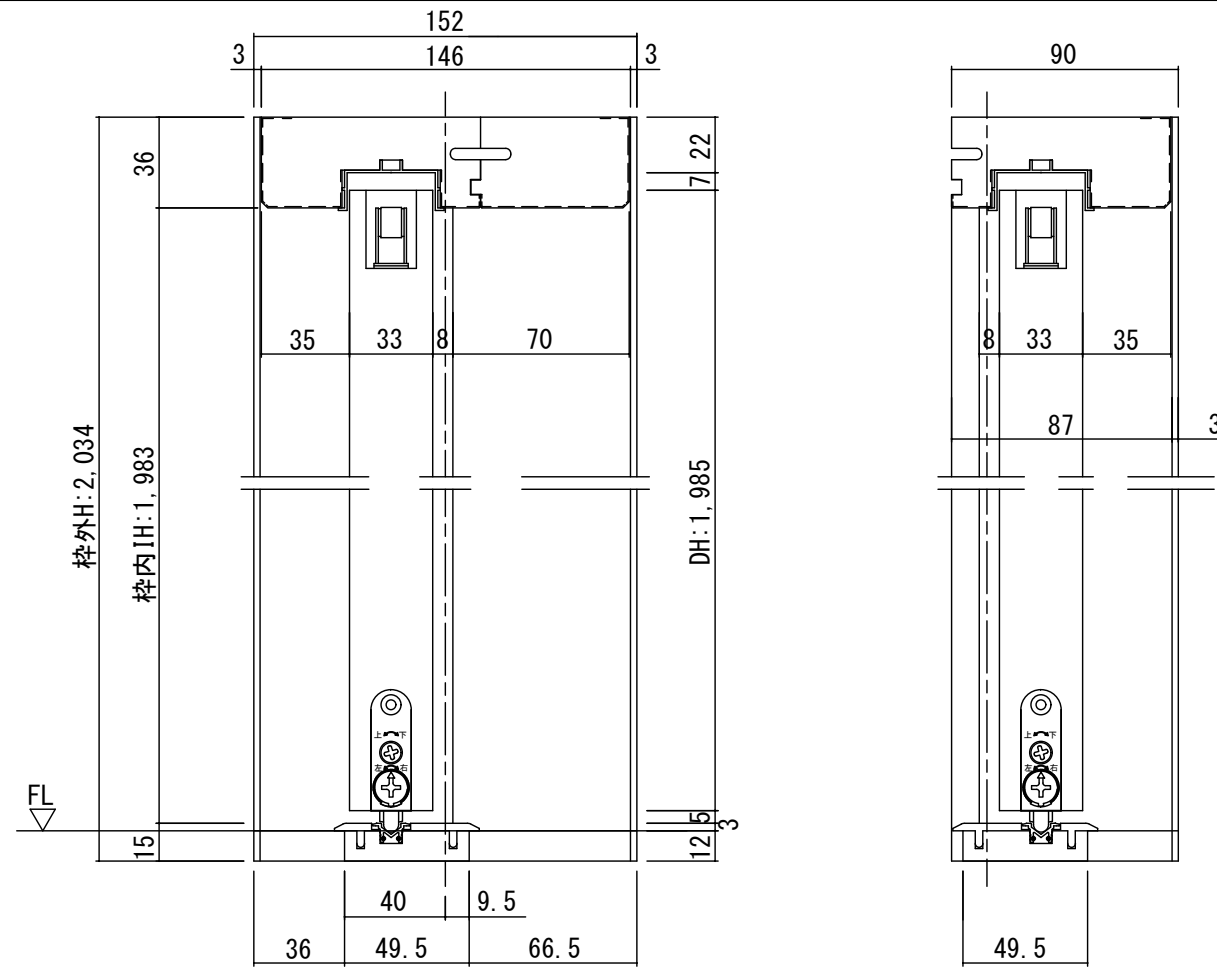
断面図
