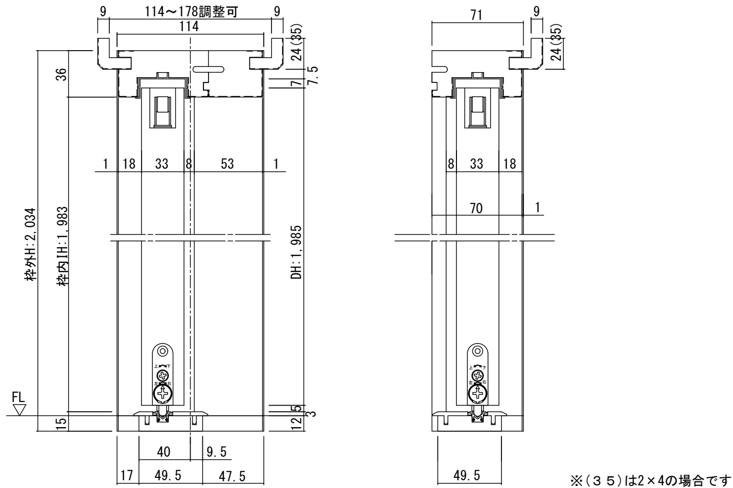
断面図
