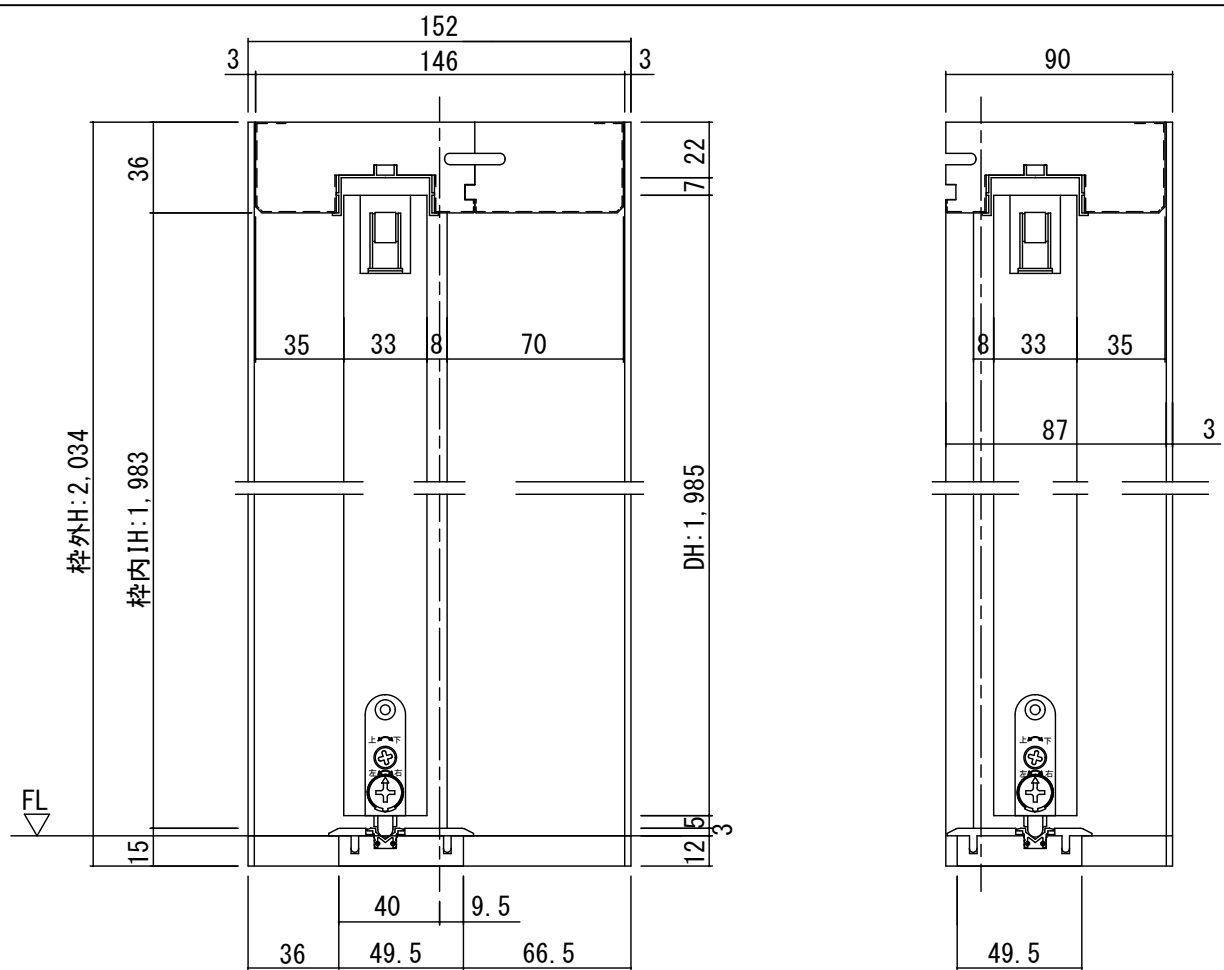
断面図
