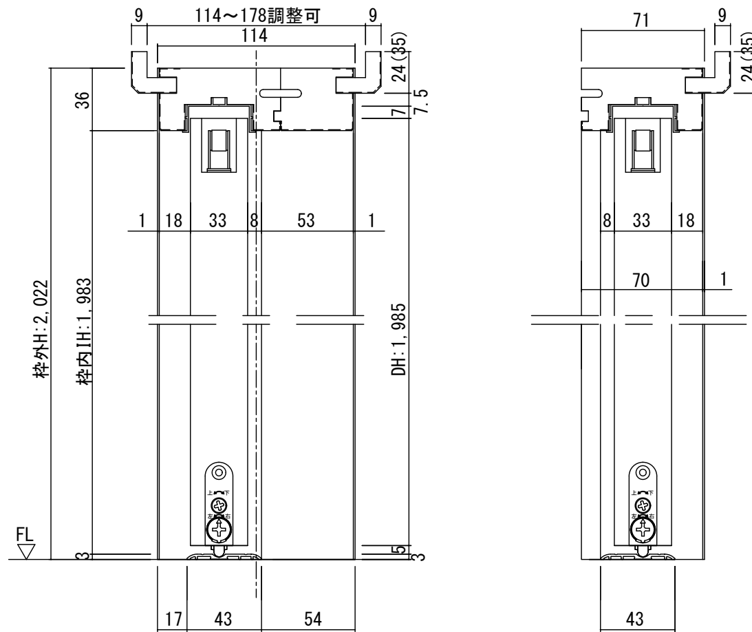
断面図
