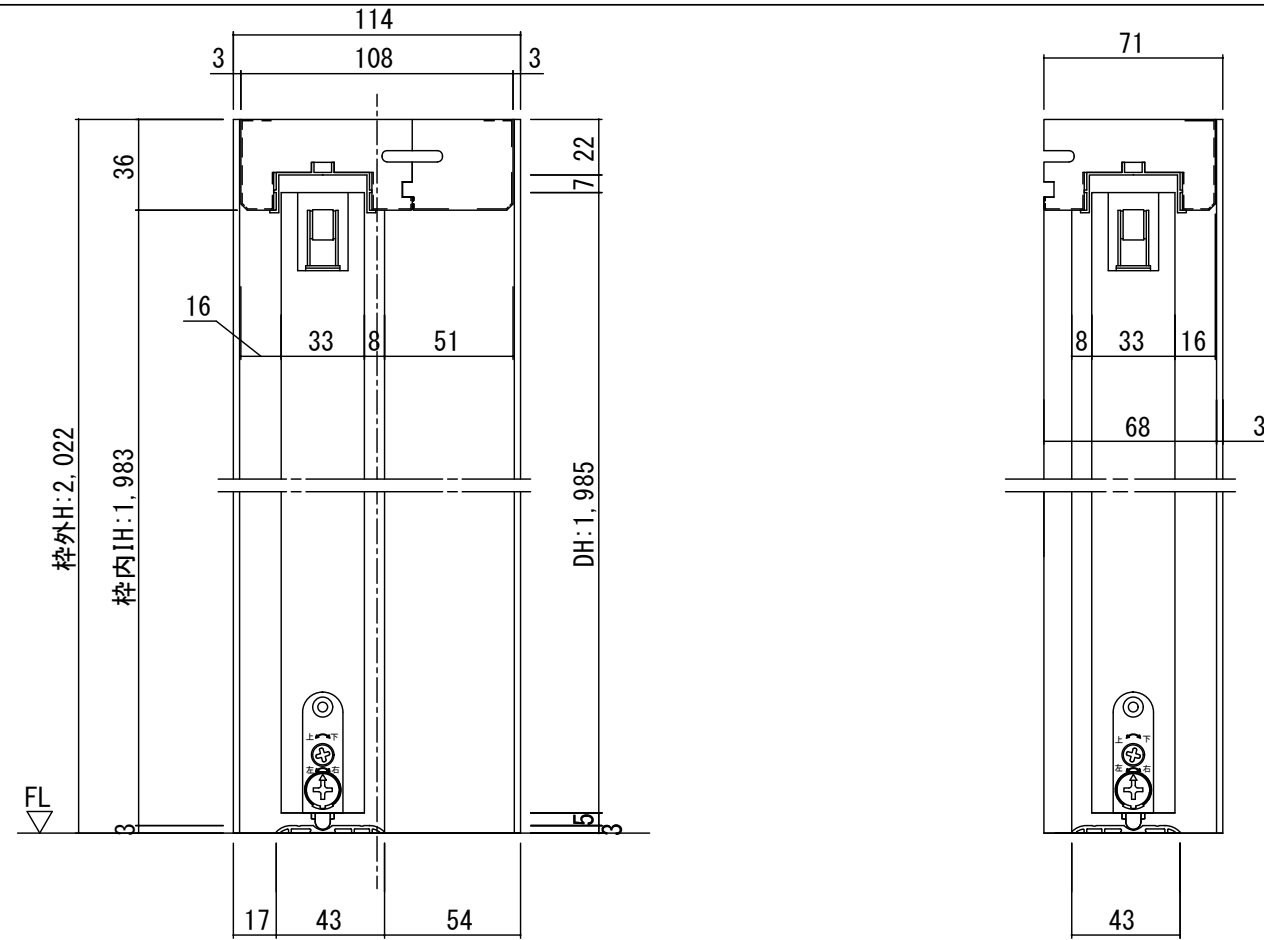
断面図
