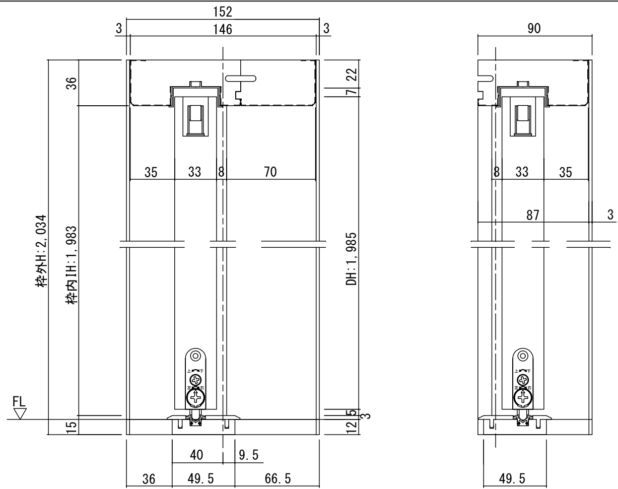
断面図
