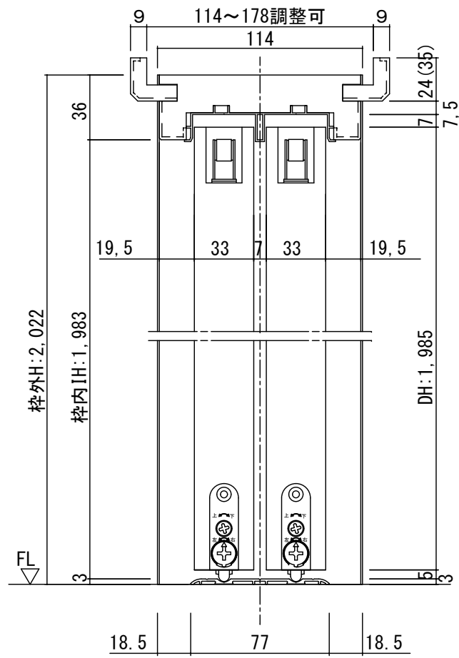
断面図
