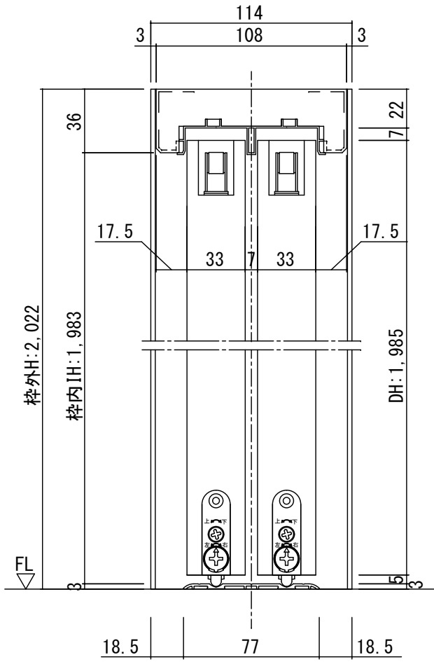
断面図
