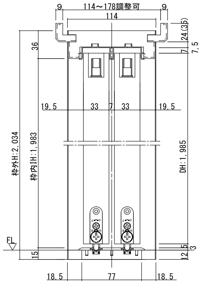
断面図
