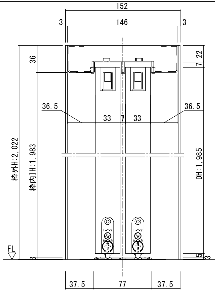
断面図
