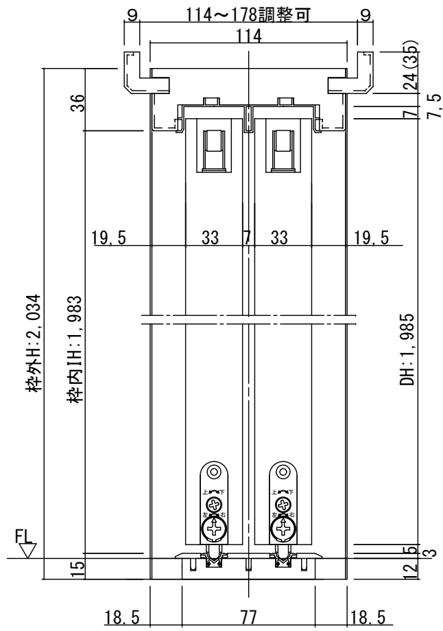
断面図
