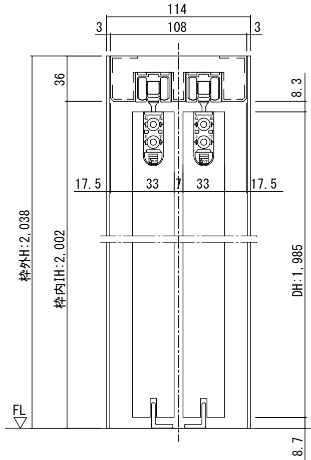
断面図
