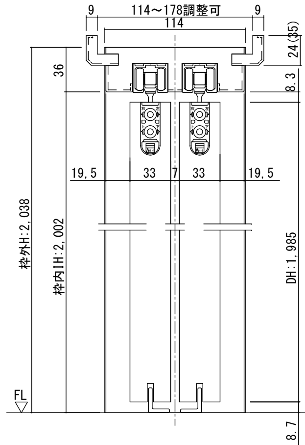
断面図
