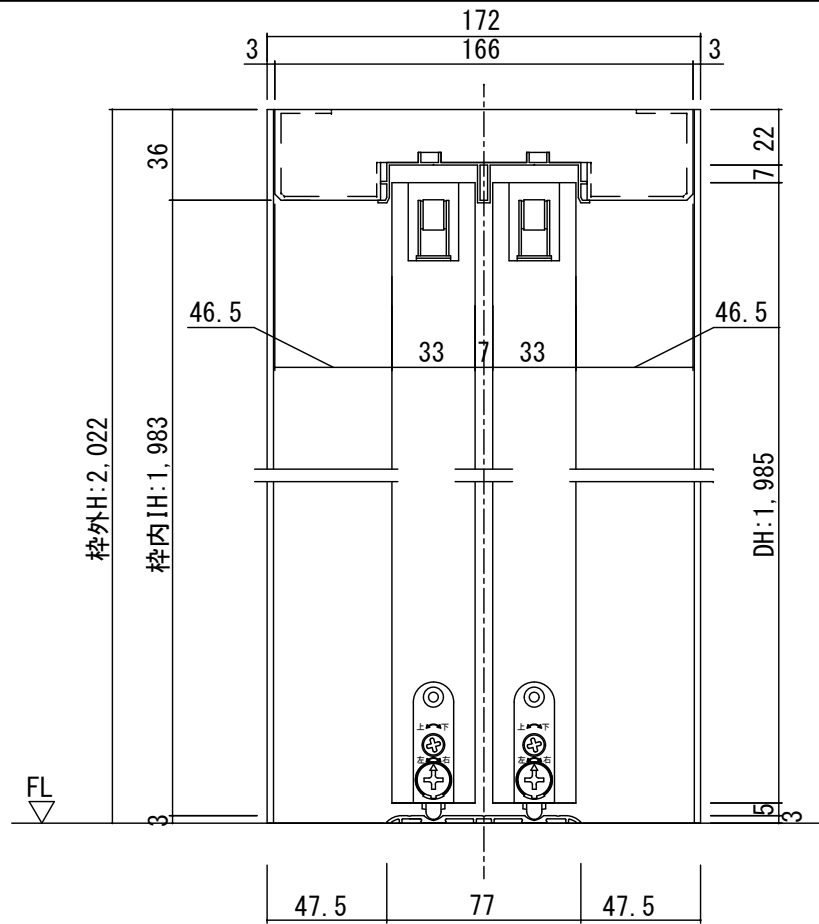
断面図
