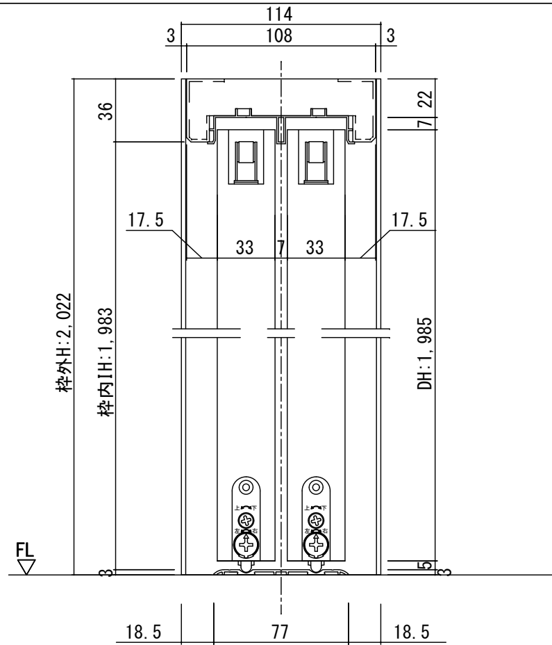
断面図
