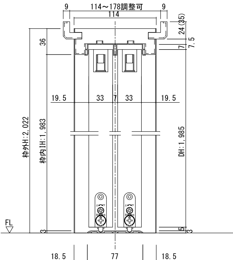
断面図
