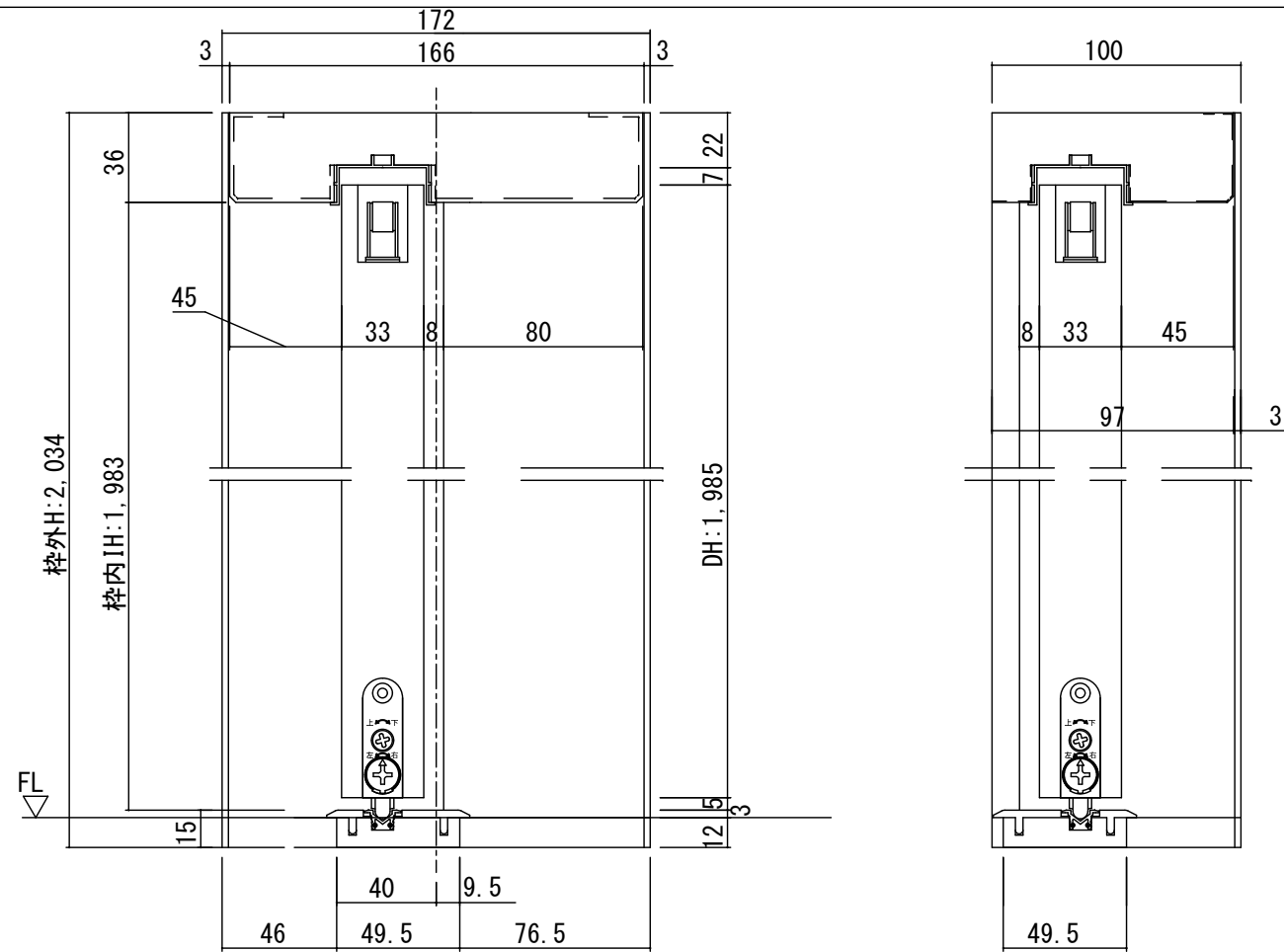
断面図
