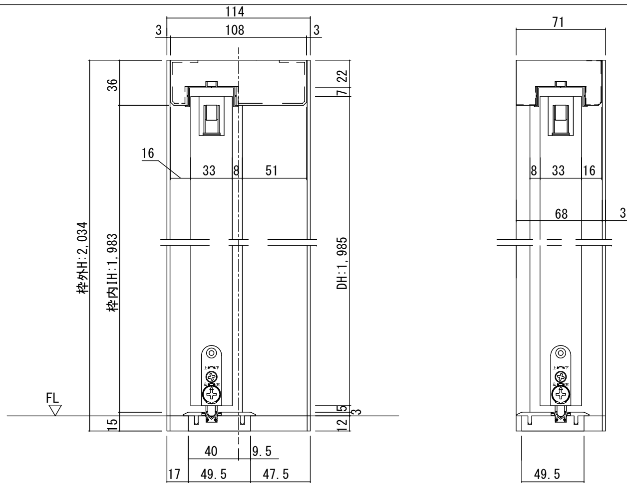
断面図
