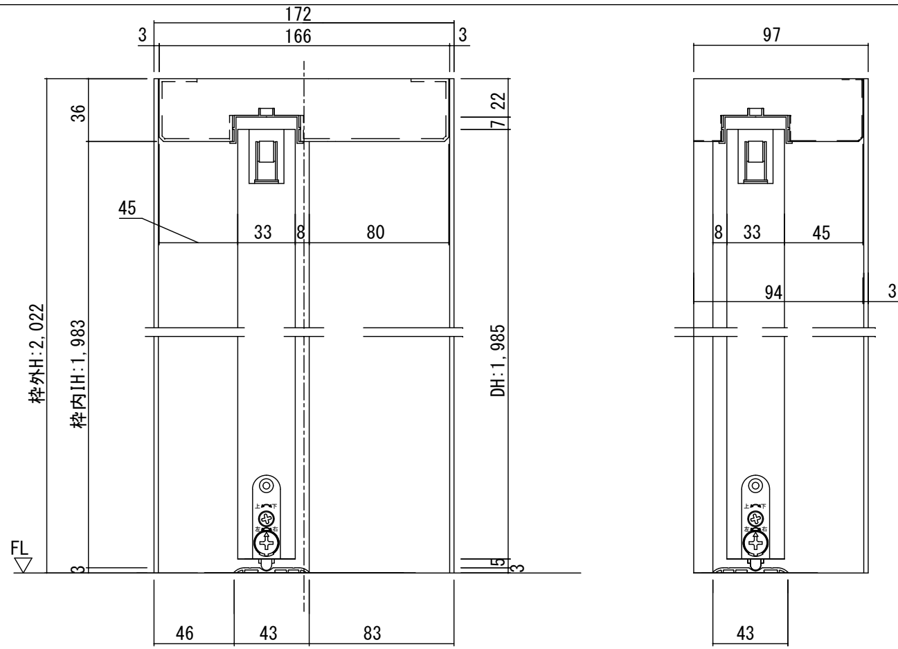
断面図
