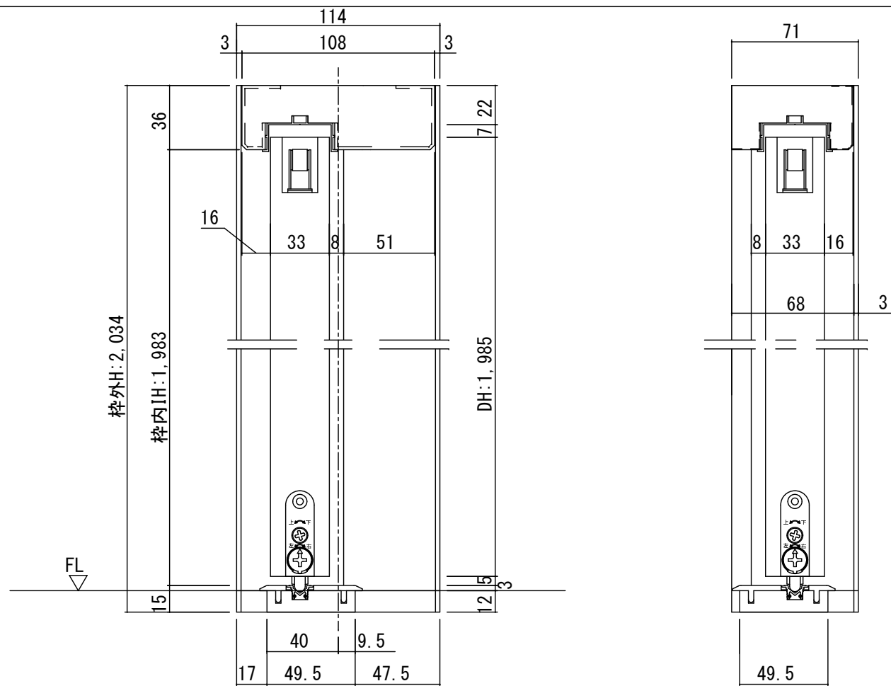
断面図
