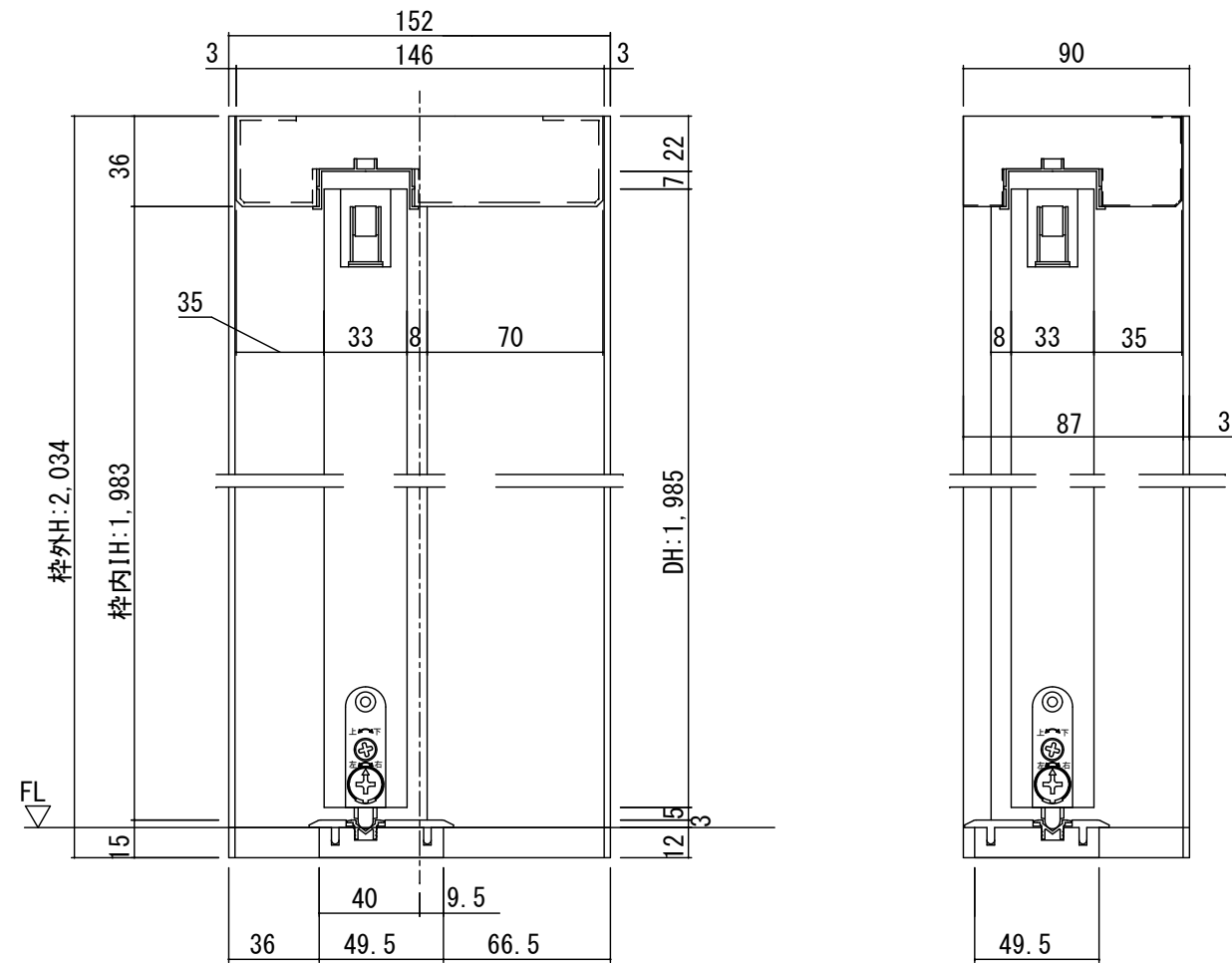
断面図
