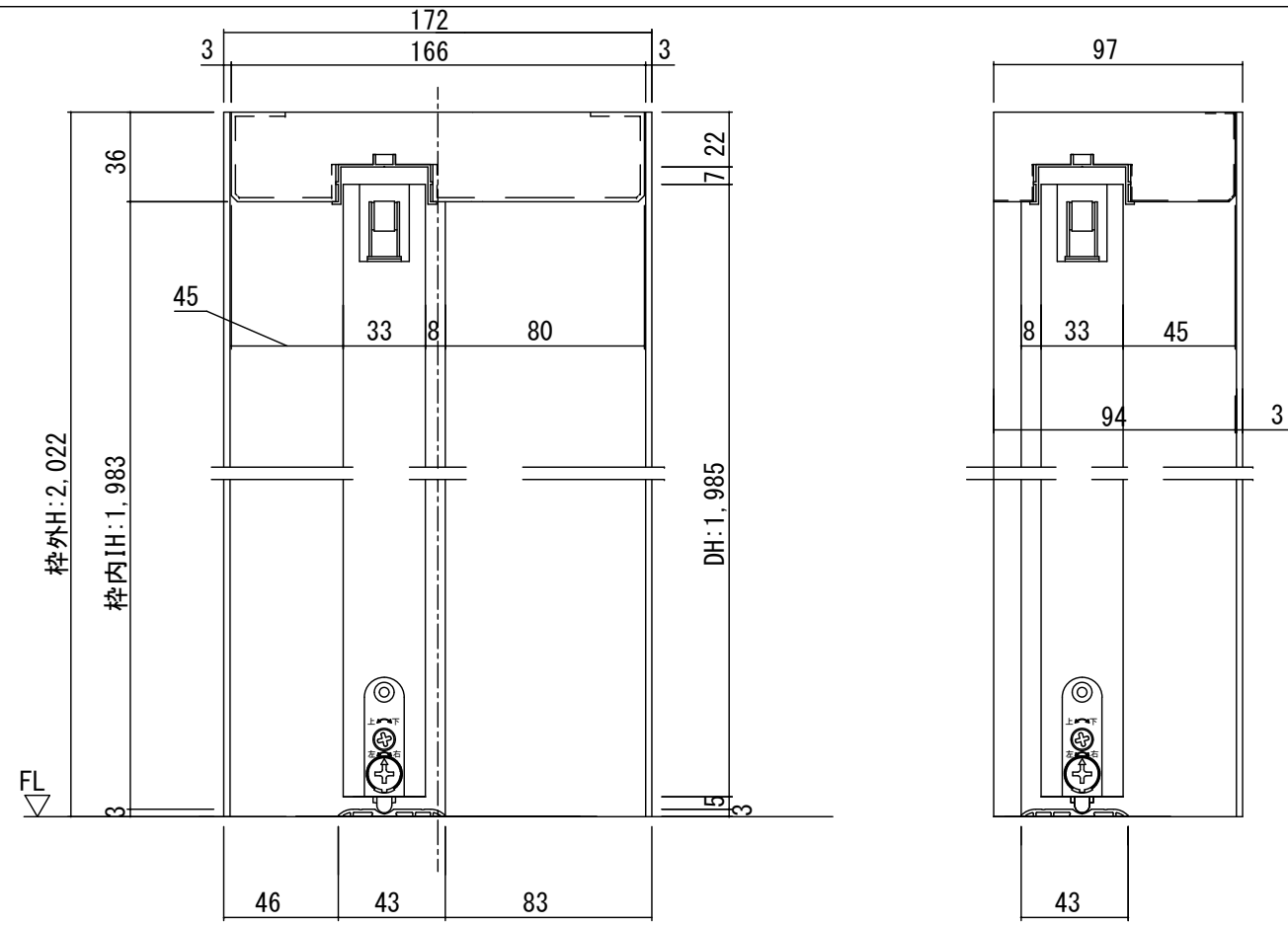
断面図
