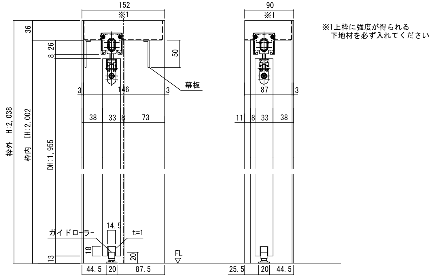
断面図
