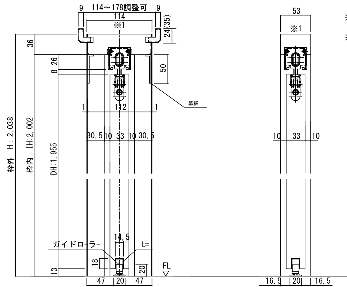
断面図
