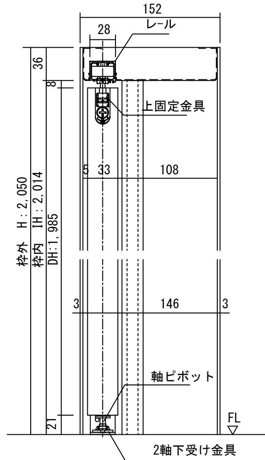
断面図
