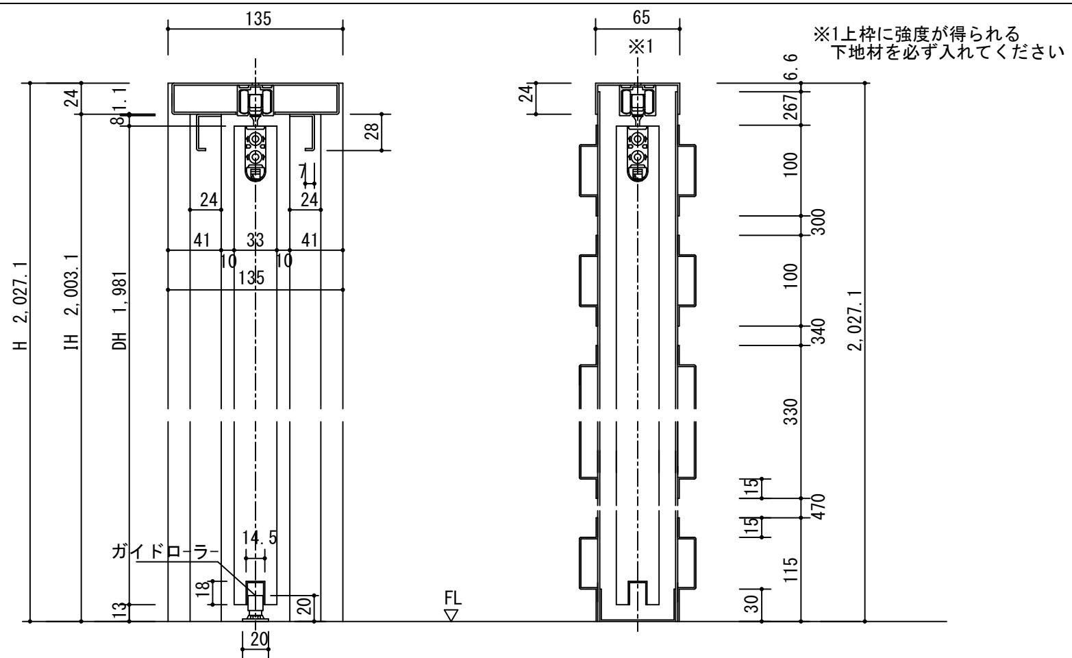
断面図
