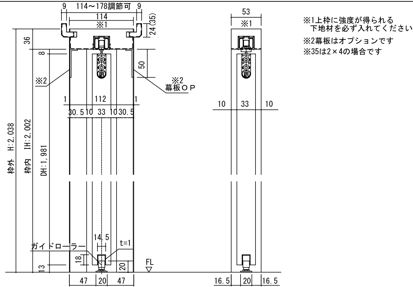
断面図
