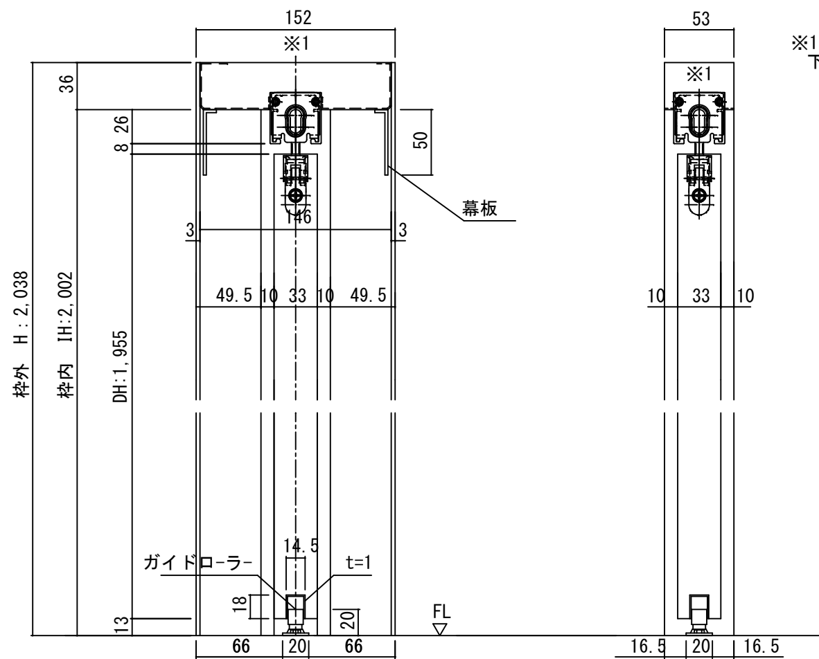
断面図
