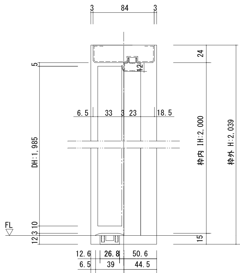
断面図
